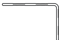
Alu-Leiste ungelocht Breite 25 mm Höhe 52 mm
