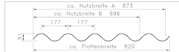
Wellprofil 177 / 51, 5-er Welle Stärke 1,2 mm. Farbe: glashell, natur transparent
