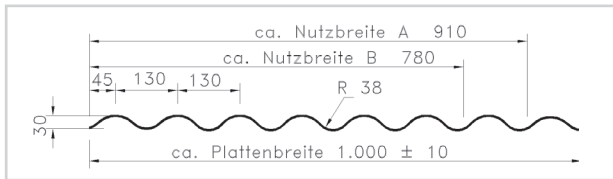
Wellprofil 130 / 30, 8er Welle Stärke 1,2 mm. Farbe: glashell
