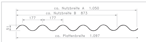
Wellprofil 177 / 51, 6-er Welle Stärke 1,2 mm. Farbe: glashell, opak grau
