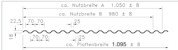
Profil Trapez 70 / 18, Stärke 1,2 mm. Farbe: glashell, natur transp., bronze, opak grau u.
