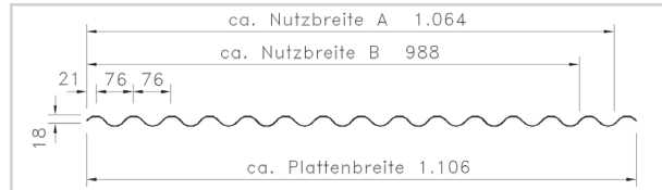
Profil Sinus 76 / 18, Stärke 1,2 mm. Farbe: glashell
